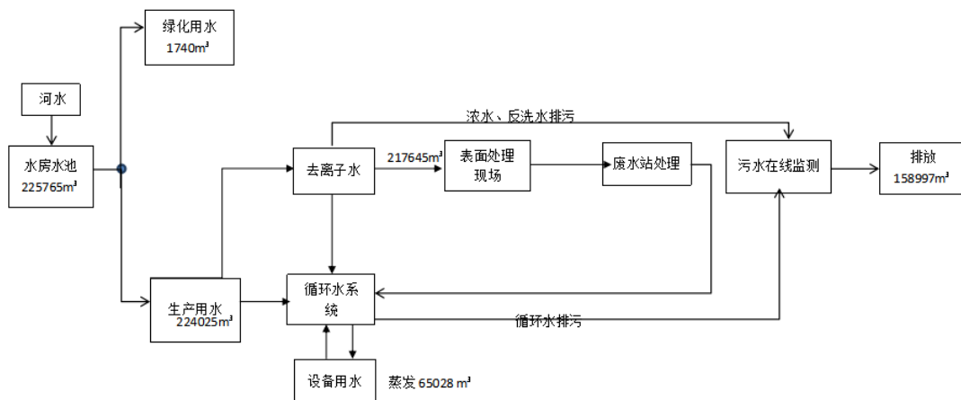
台山市金桥铝型材厂有限公司水平衡图
